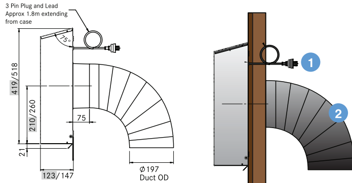
EW-765/1140 Dimensions EW-2010 Dimensions
